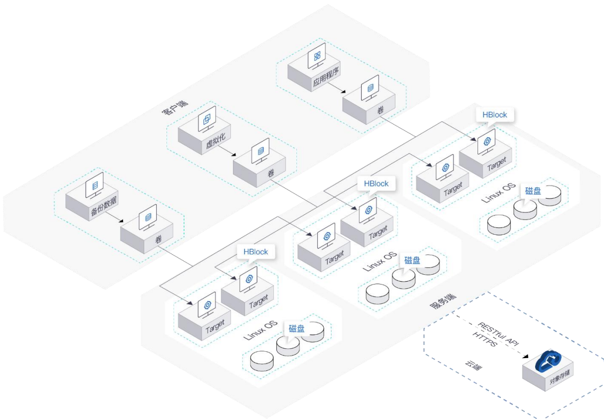
图1.HBlock 架构图
