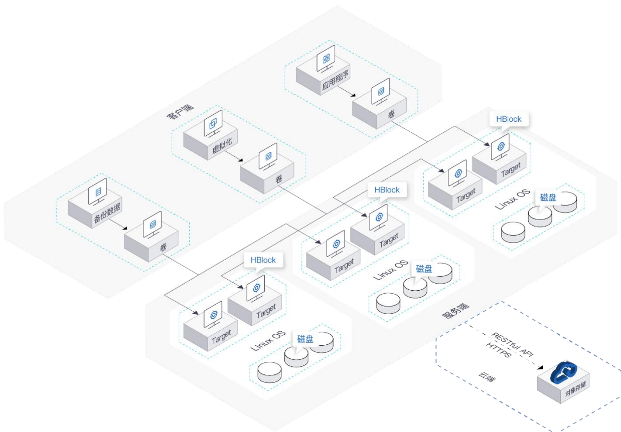
图1.HBlock 架构图
