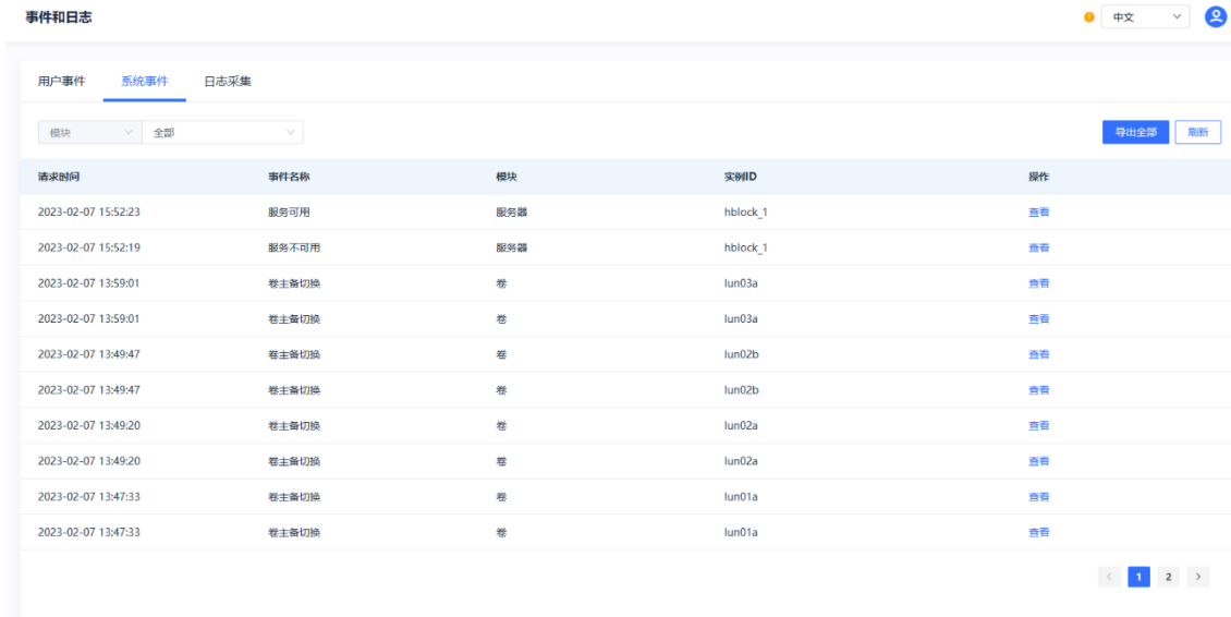
图159. 系统事件
