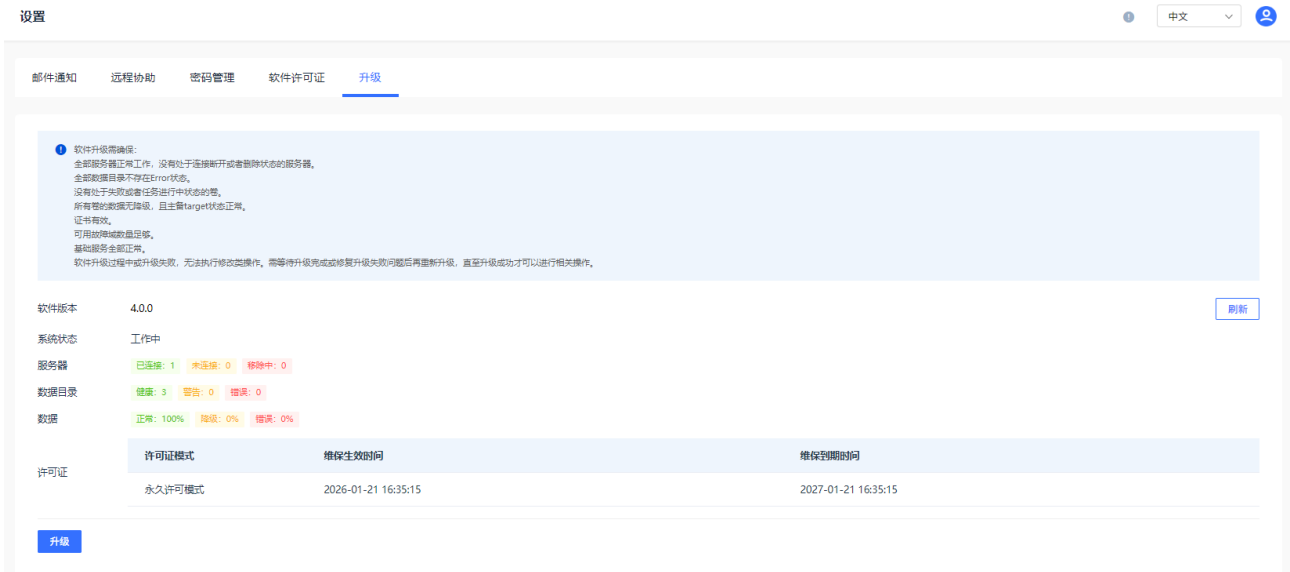
图174. 升级（单机版）
