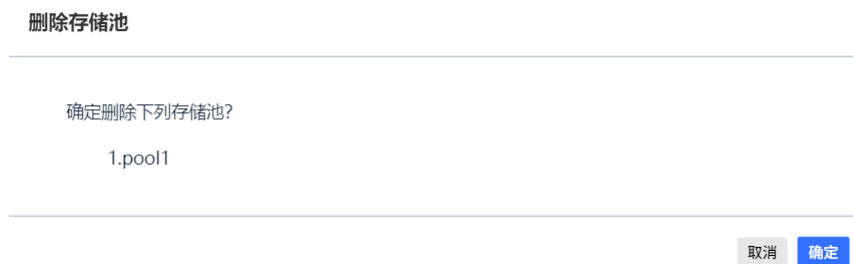
图76. 删除存储池
