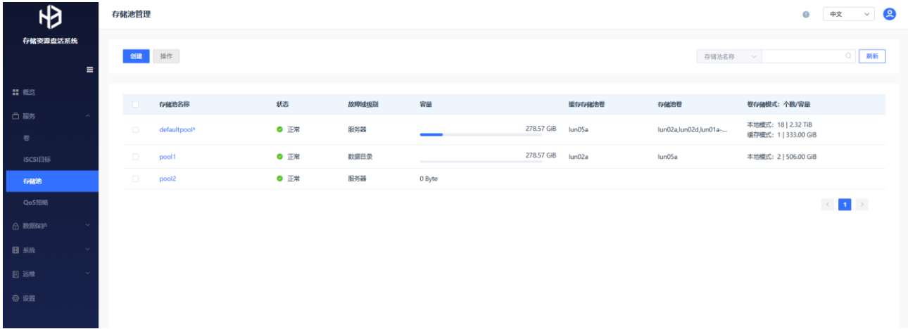
图68. 存储池管理
