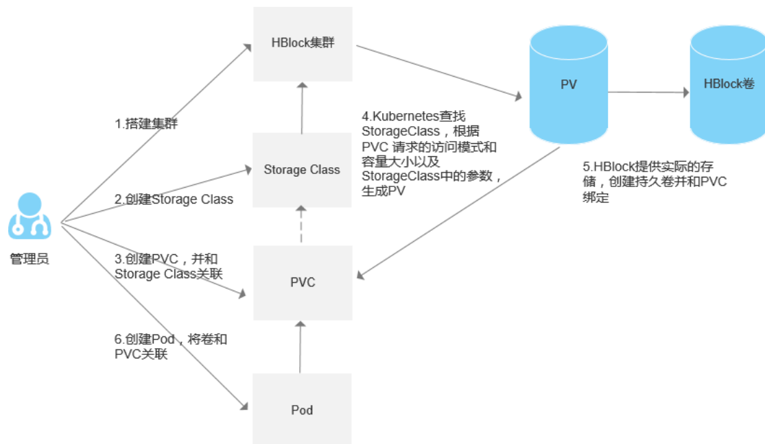
图4.动态 PV 流程图
